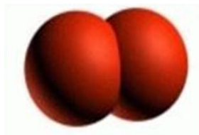
kyslík - O 2
