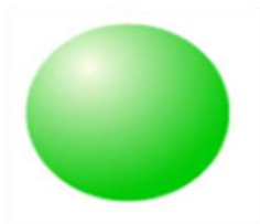
dusík - N
